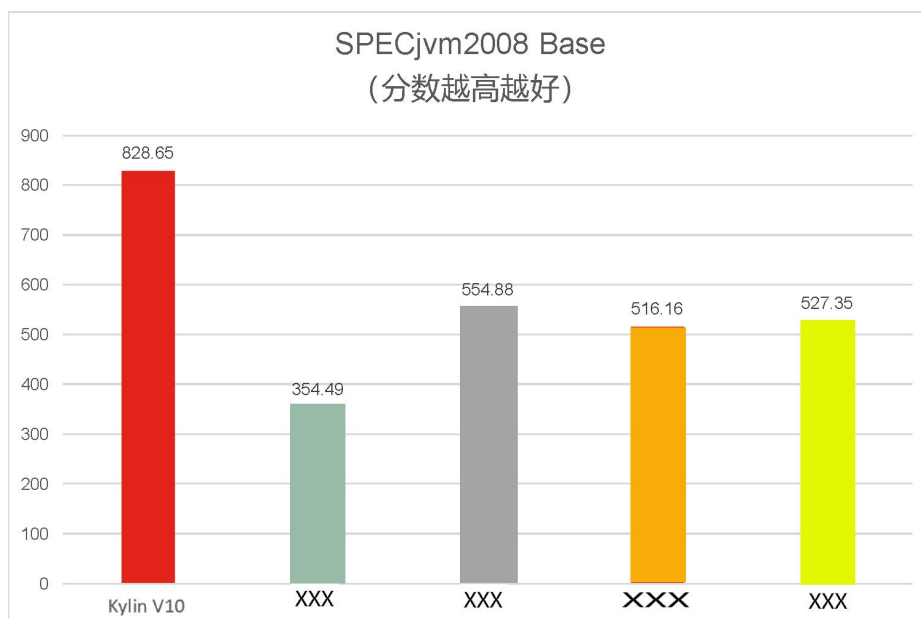
图 2-6 JRE 运行性能（java 应用场景）-SPECJVM 2008（长城 DF720）
