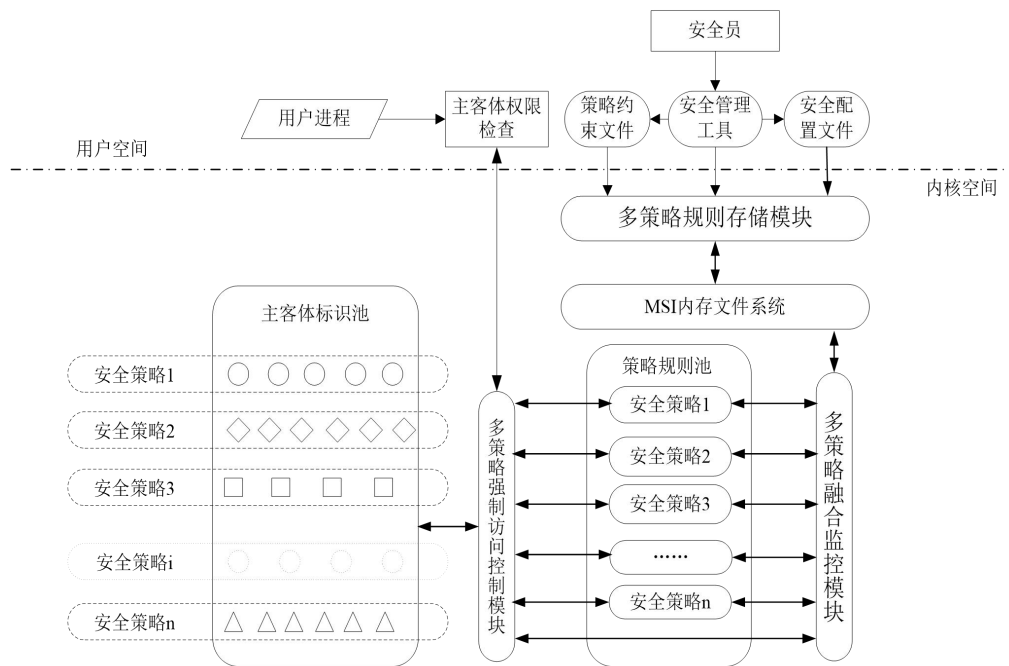
图 2-9 多策略融合控制总体流程
