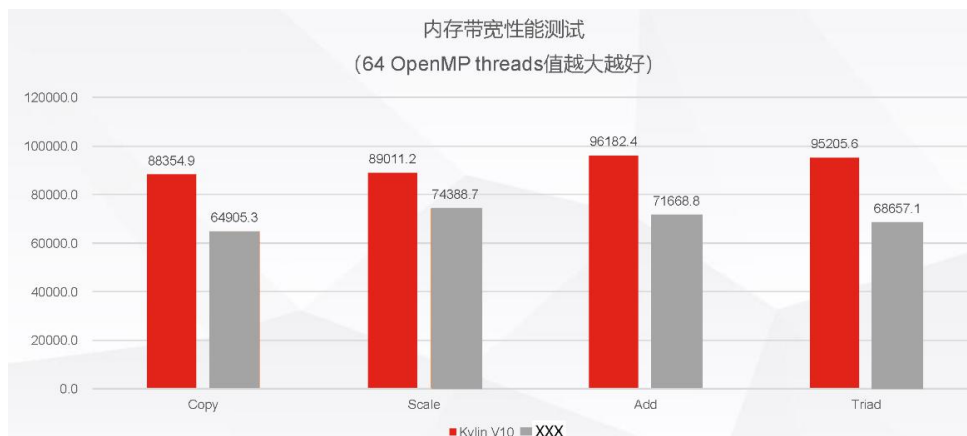
图 2-7 内存带宽性能测试-64 OpenMP threads（长城 DF720）
