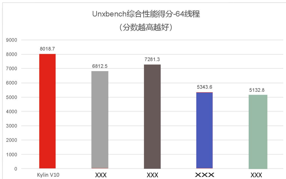
图 2-4 Unixbench 综合性能测试-64 线程（长城 DF720）
