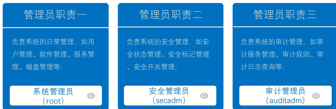
图 2-12 管理员分权
