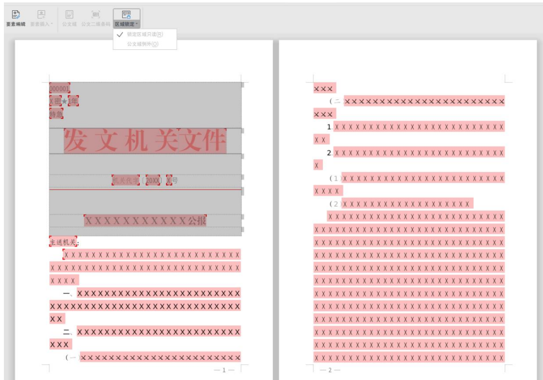
图 2.2.18.11 区域锁定
