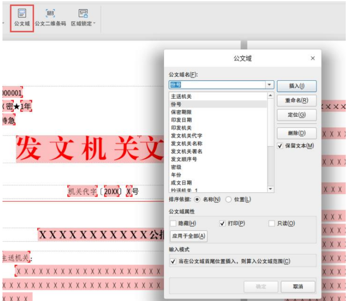
图 2.2.18.10 公文域
