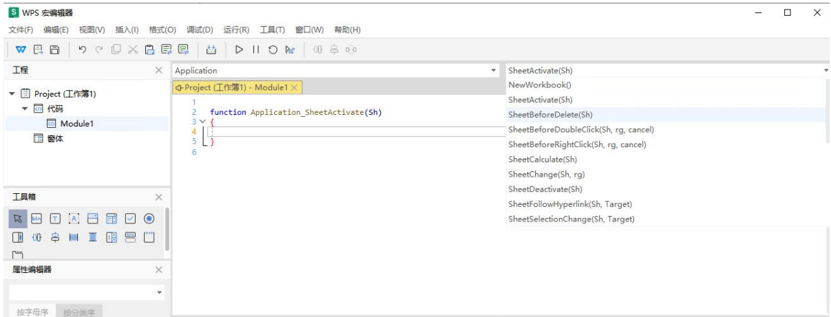
图 3.1.1-2 对象导航栏
