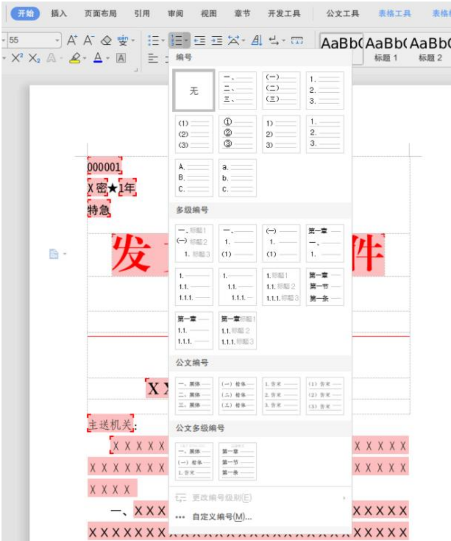
图 2.2.18.13 公文编号
