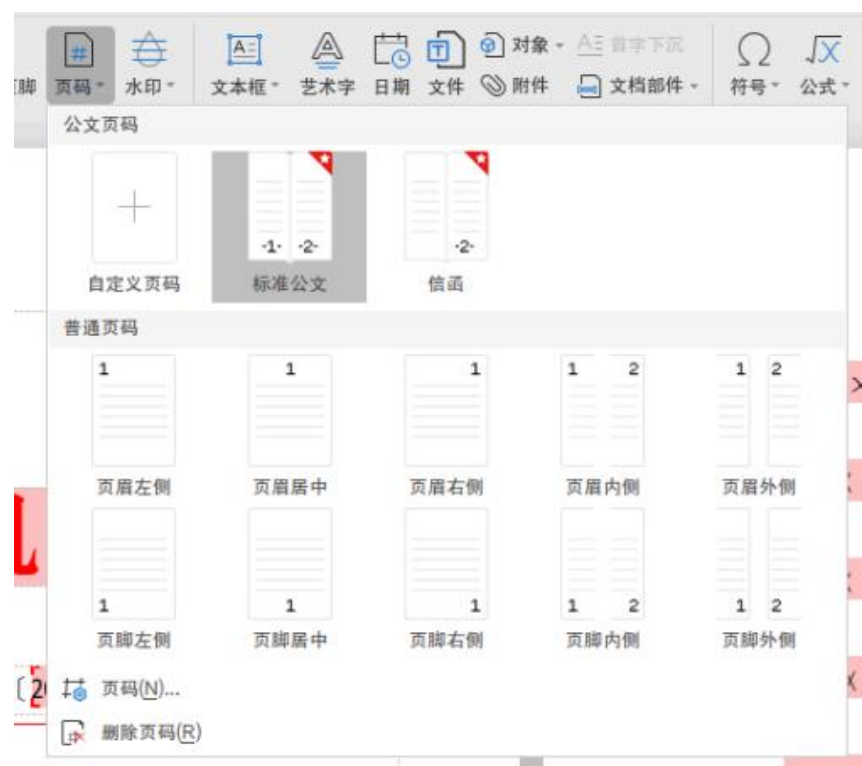
图 2.2.18.15-1 公文页码
