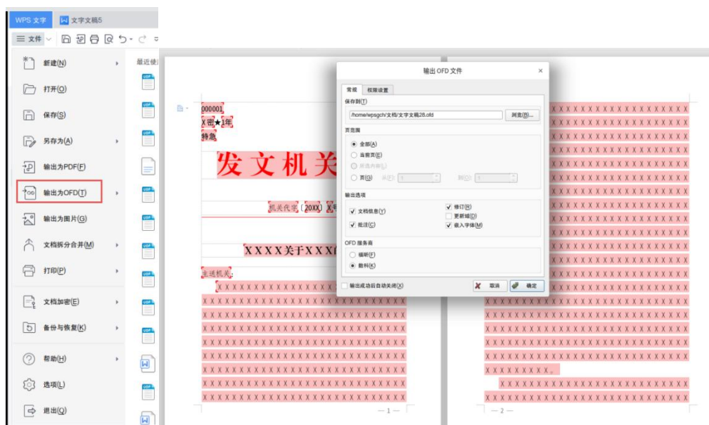
图 2.2.18.23-2 输出为 OFD
