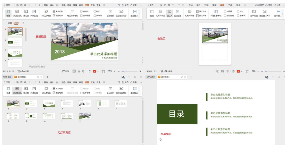
图 2.3-9-2 视图展示
