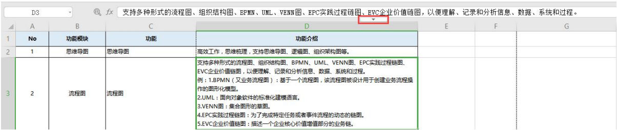
图 2.4.7 智能收缩
