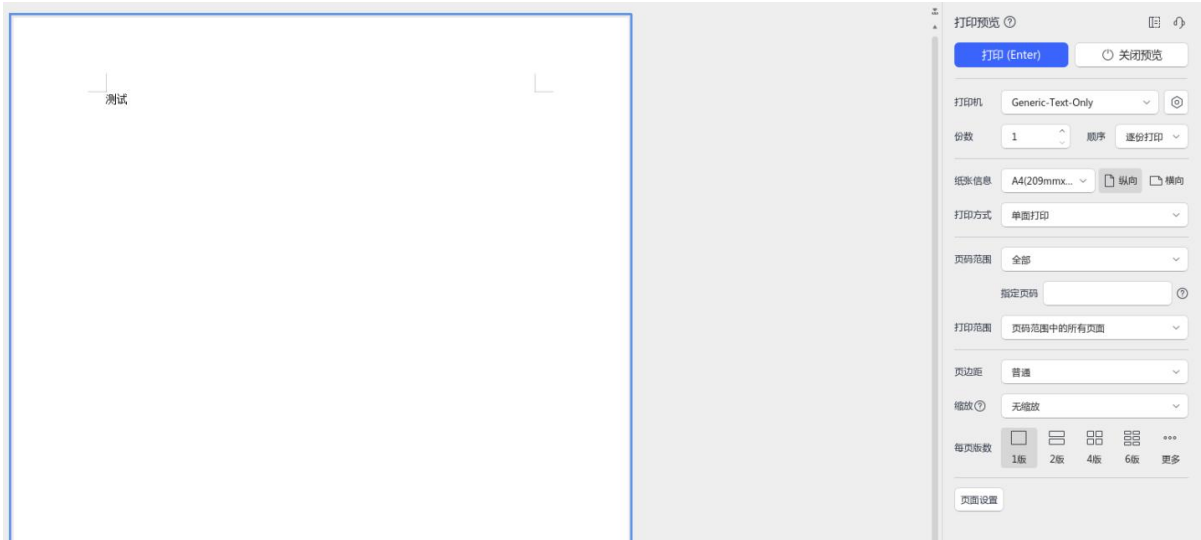
图 2.1.10 打印
