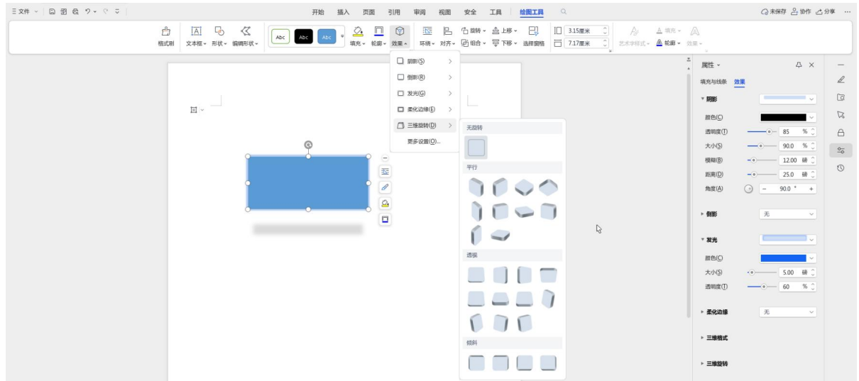
图 2.1.8 设置三维
