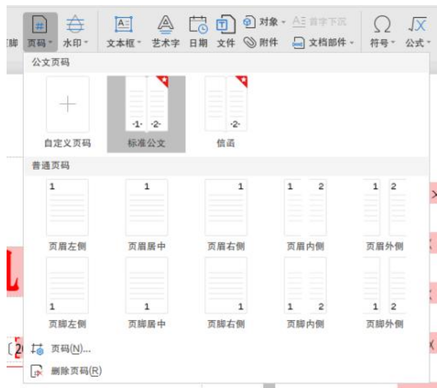
图 2.2.18.15-1 公文页码
