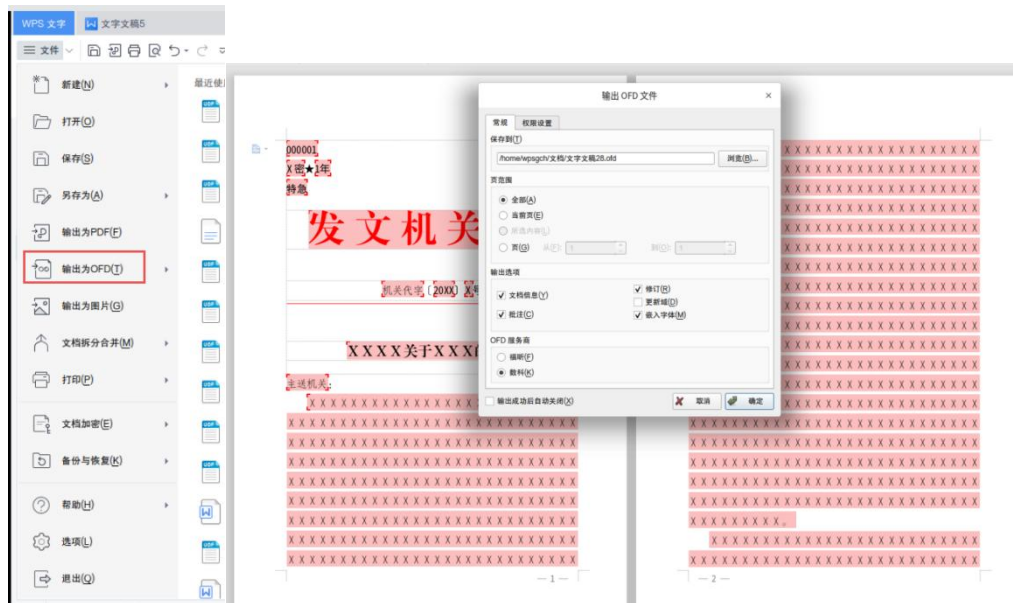
图 2.2.18.23-2 输出为 OFD
