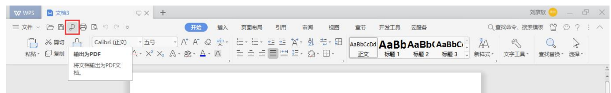
图 2.1.2 输出为 PDF
