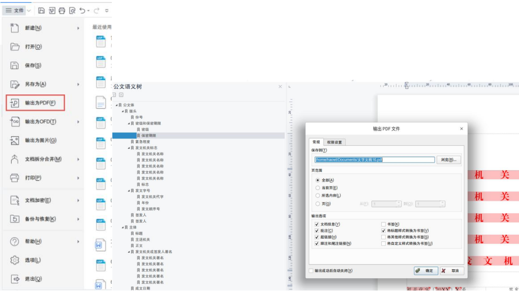
图 2.2.18.23-1 输出为 PDF
