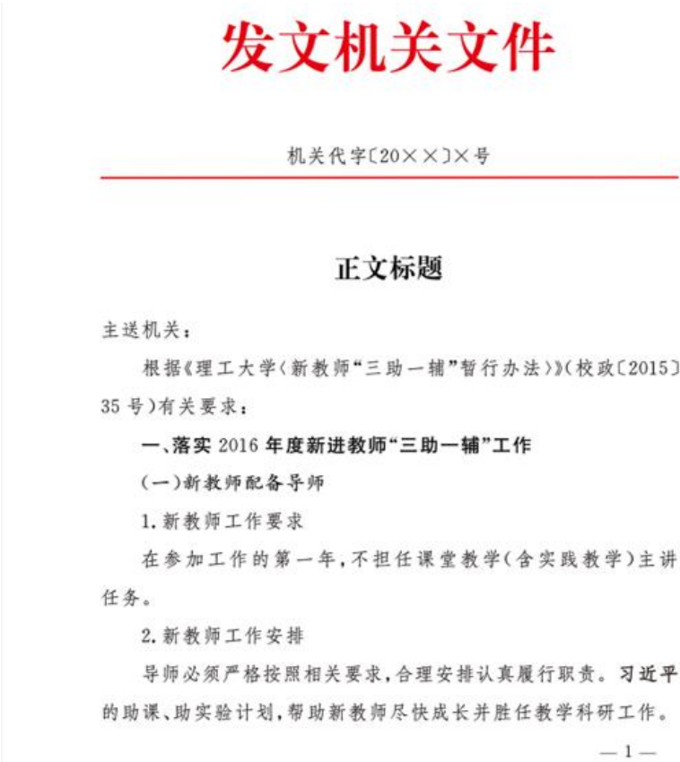
图 2.2.18.24 公文打印
